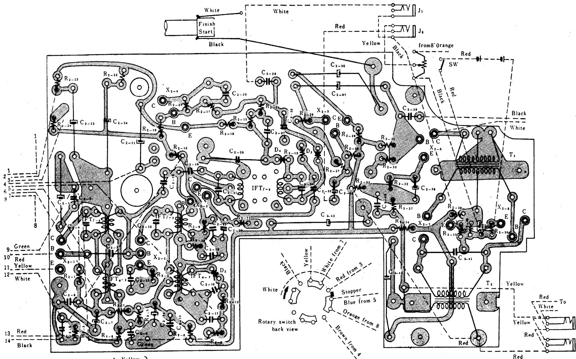
CIRCUITO STAMPATO delle SEZIONI MEDIA F. e B.F. del TFM-121
